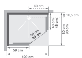
Installations réversibles gauche / droite
