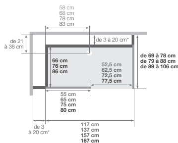
Installation réversible gauche/droite
