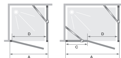
Tailles ≤ 100 cm Tailles ≥ 120 cm Montage en angle avec Smart Express+ Fixe Installation réversible gauche / droite
