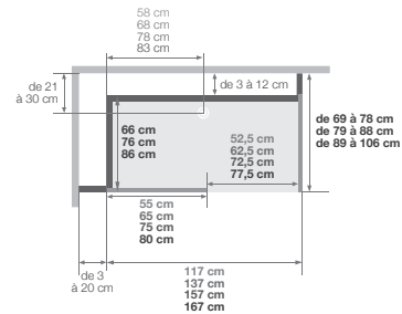
Installation réversible gauche/droite
