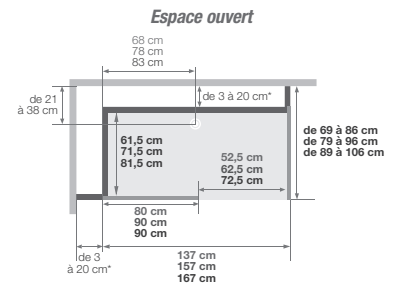
Version haute en angle Installations réversibles gauche / droite
