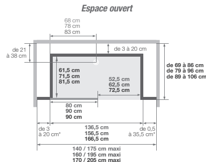
Version haute en niche Installations réversibles gauche / droite
